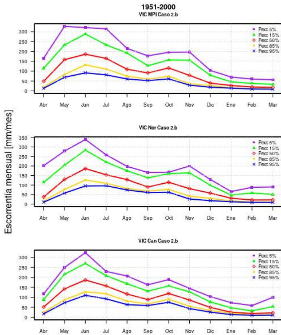
Figura A.16: Curva de variación estacional caso 2.b para modelos MPI, Nor y Can entre 1951 y 2000.
