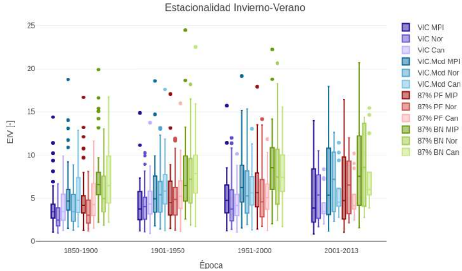
Figura 5.10: Gráfico de cajas de índice de estacionalidad invierno-verano en simulaciones de casos 0, 1, 2.a y 2.b, para los MCG MPI, Nor y Can, entre 1850 y 2013 para cuenca del Río Bío Bío.
