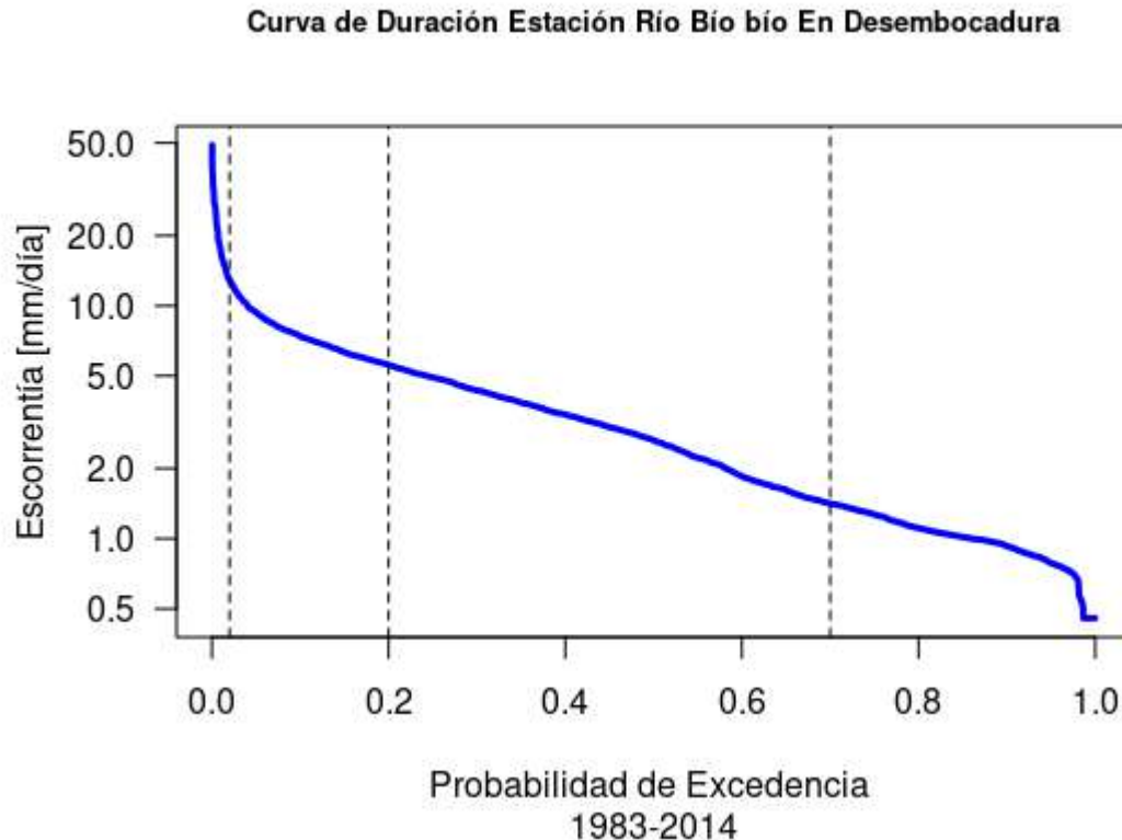
Figura 3.4: Curva de duración de caudales diarios entre 1983 y 2014 para la Río Bío bío En Desembocadura. Fuente: DGA.
