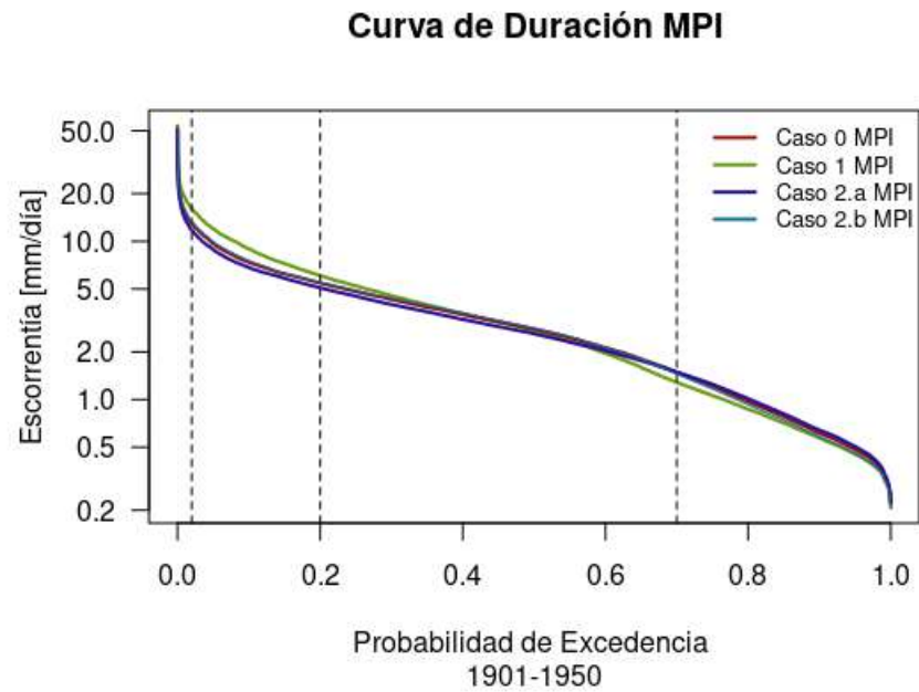
Figura A.23: Curva de duración para casos 0, 1, 2.a y 2.b entre 1901 y 1950 modelo MPI.
