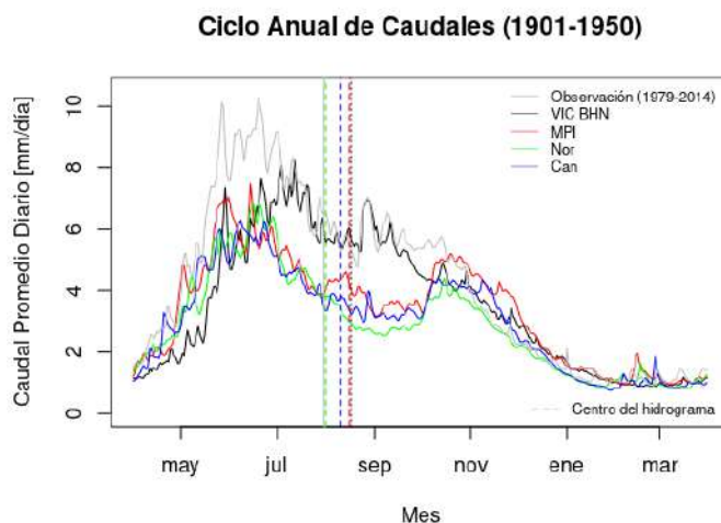
Figura A.19: Ciclo de caudales anuales para MPI, Nor y Can, VIC con entradas de BHN y Observaciones entre 1901 y 1950 para la cuenca del río Bío bío.
