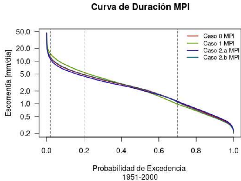
Figura A.24: Curva de duración para casos 0, 1, 2.a y 2.b entre 1951 y 2000 modelo MPI.
