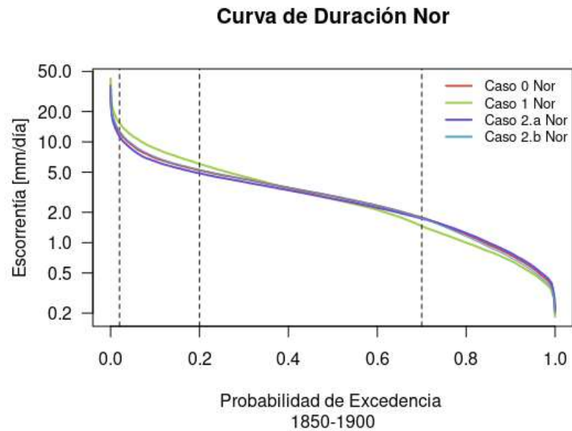
Figura A.26: Curva de duración para casos 0, 1, 2.a y 2.b entre 1850 y 1900 modelo Nor.
