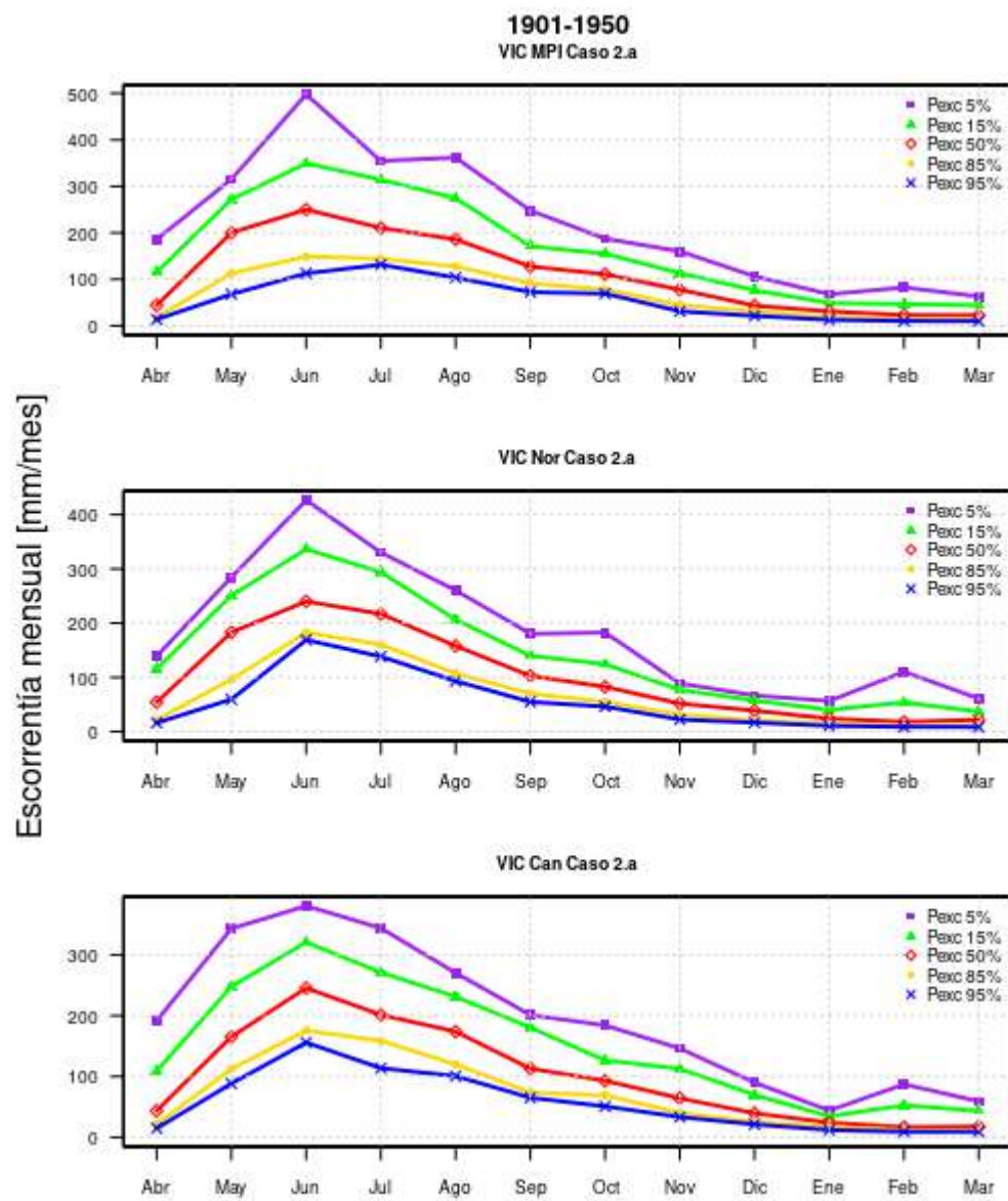
Figura A.11: Curva de variación estacional caso 2.a para modelos MPI, Nor y Can entre 1901 y 1950.
