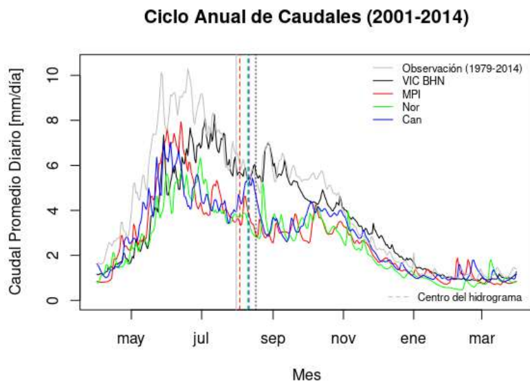
Figura 5.19: Ciclo anual de caudales para caso 0 utilizado MPI, Nor y Can entre 2001 y 2014.
