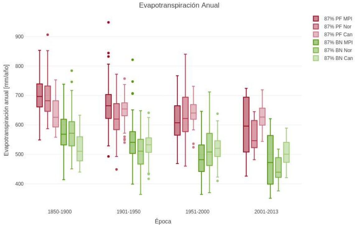
Figura 5.22: Gráfico de cajas de evapotranspiración anual obtenida en simulaciones de casos 2.a y 2.b, para los MCG MPI, Nor y Can, entre 1979 y 2014 para cuenca del Río Bío Bío.
