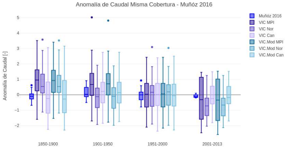
Figura 5.4: Gráfico de cajas de anomalías de caudal para serie dendrocronológica y simulaciones de casos 0 y 1 entre 1979 y 2014 para cuencas en régimen natural utilizadas en Muñoz et al. ,2016.
