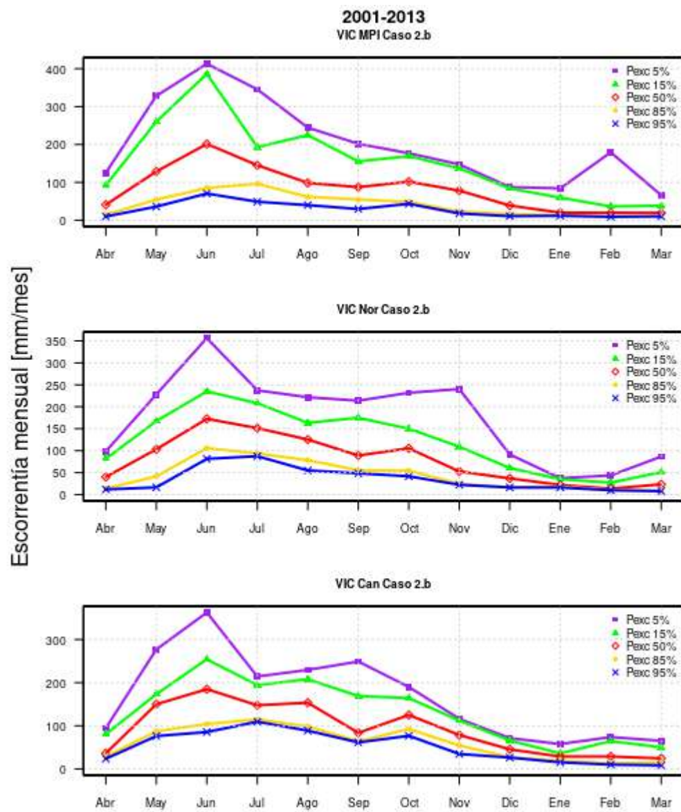
Figura A.17: Curva de variación estacional caso 2.b para modelos MPI, Nor y Can entre 2001 y 2013.
