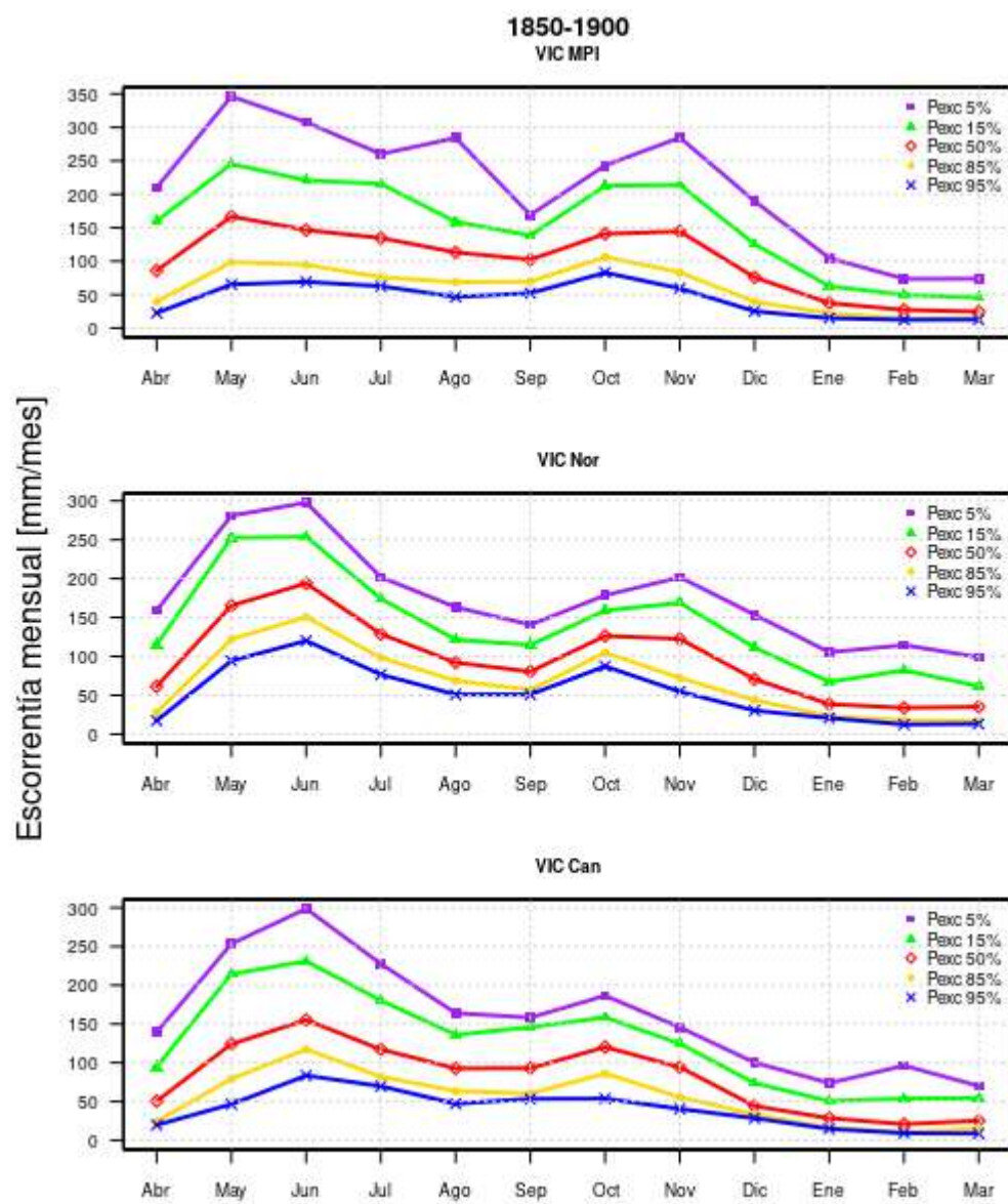
Figura A.2: Curva de variación estacional caso 0 para modelos MPI, Nor y Can entre 1850 y 1900.
