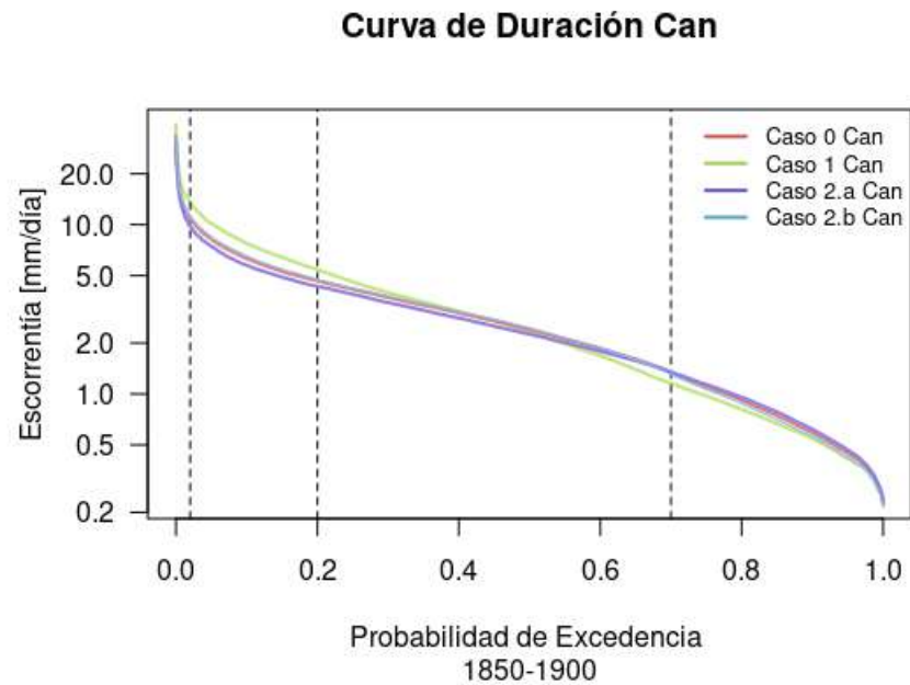
Figura A.30: Curva de duración para casos 0, 1, 2.a y 2.b entre 1850 y 1900 modelo Can.
