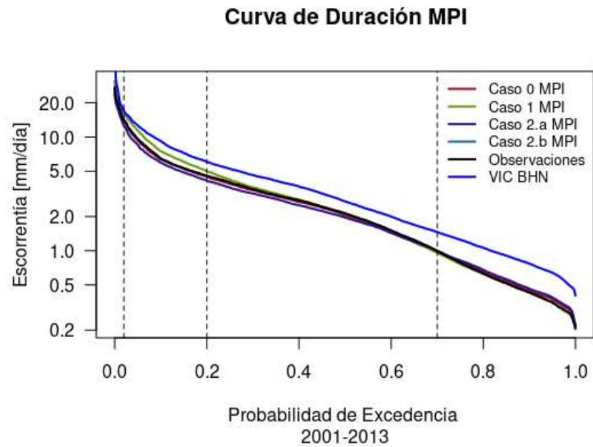
Figura A.25: Curva de duración para casos 0, 1, 2.a y 2.b entre 2001 y 2013 modelo MPI.
