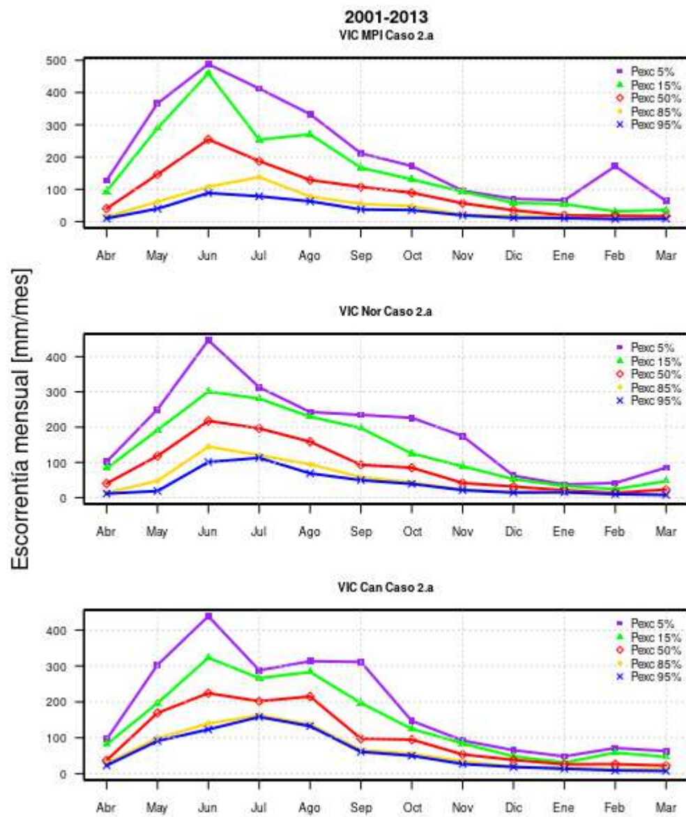
Figura A.13: Curva de variación estacional caso 2.a para modelos MPI, Nor y Can entre 2001 y 2013.
