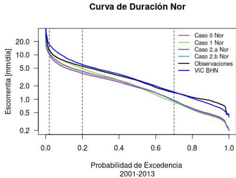
Figura A.29: Curva de duración para casos 0, 1, 2.a y 2.b entre 2001 y 2013 modelo Nor.
