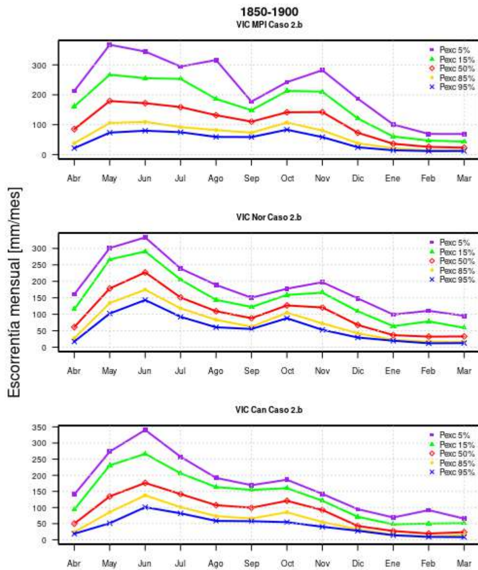
Figura A.14: Curva de variación estacional caso 2.b para modelos MPI, Nor y Can entre 1850 y 1900.
