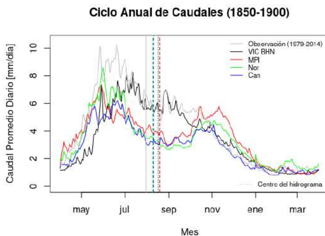
Figura A.18: Ciclo de caudales anuales para MPI, Nor y Can, VIC con entradas de BHN y Observaciones entre 1850 y 1900 para la cuenca del río Bío bío.
