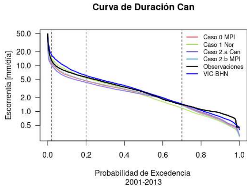
Figura A.33: Curva de duración para casos 0, 1, 2.a y 2.b entre 2001 y 2013 modelo Can.
