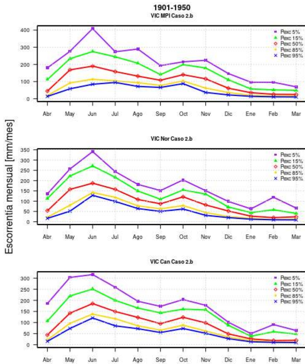
Figura A.15: Curva de variación estacional caso 2.b para modelos MPI, Nor y Can entre 1901 y 1950.
